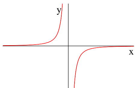
neomeđena funkcija
