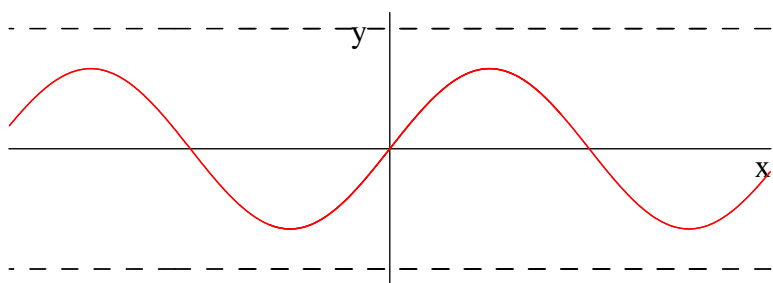
omeđena funkcija
